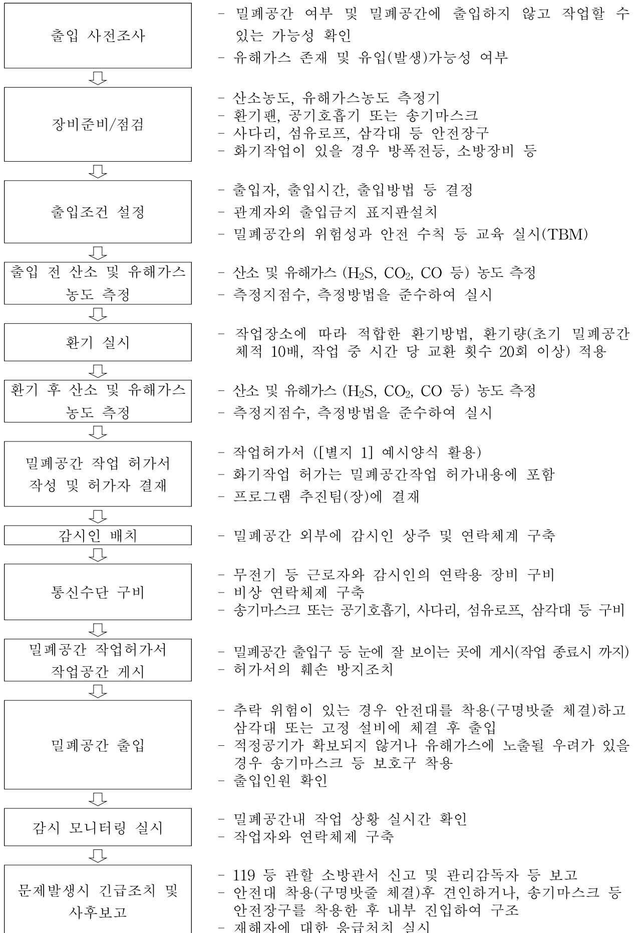
<그림 4> 밀폐공간 작업의 절차
