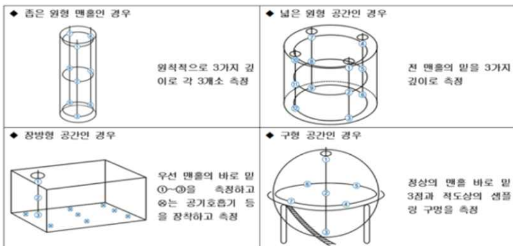
<그림 5> 밀폐공간 내 산소 및 유해가스 농도 측정 방법
